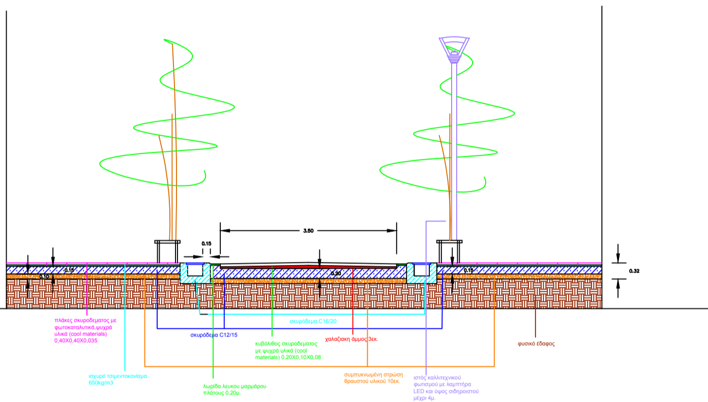
ΤΟΜΗ Α-Α ΟΔΟΣ ΜΕΡΛΟΠΟΥΛΟΥ
